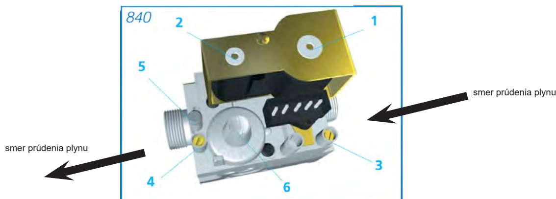
12. obrázok: Meracie výstupy na meranie tlaku plynu EMV SIT
