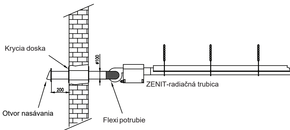
10. obrázok: Zásobovanie vzduchom k spaľovaniu z vonkajšieho priestoru
