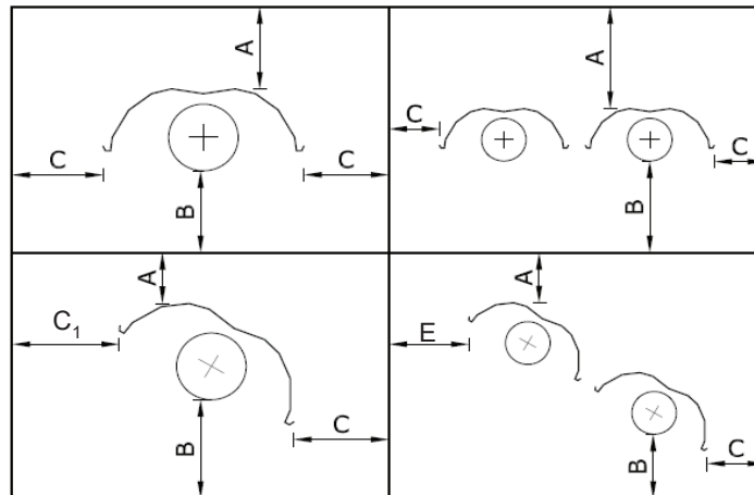
6. obrázok: Protipožiarne vzdialenosti
