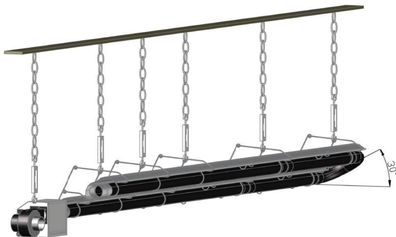
8. obrázok: Maximálny uhol sklonu pri inštalácii
