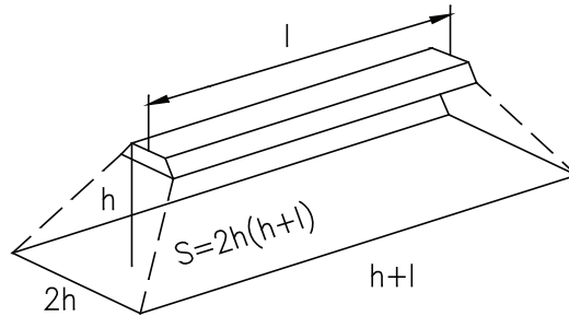
5. obrázok: Schéma oblasti osálenia povrchu
