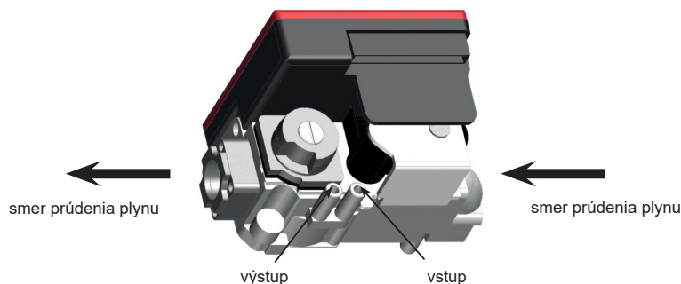
11. obrázok: Meracie výstupy na meranie tlaku plynu EMV HONEYWELL
