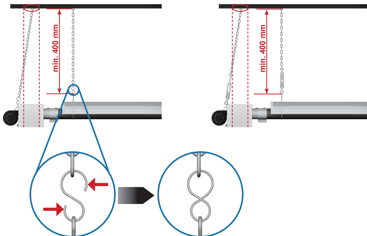
9. obrázok: Možnosti zavesenia
